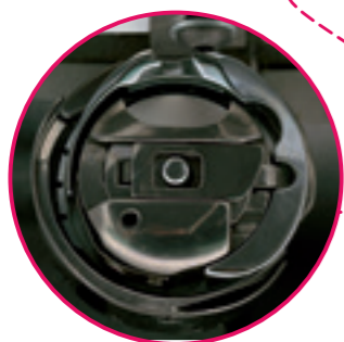
Robuster Doppelumlaufgreifer
